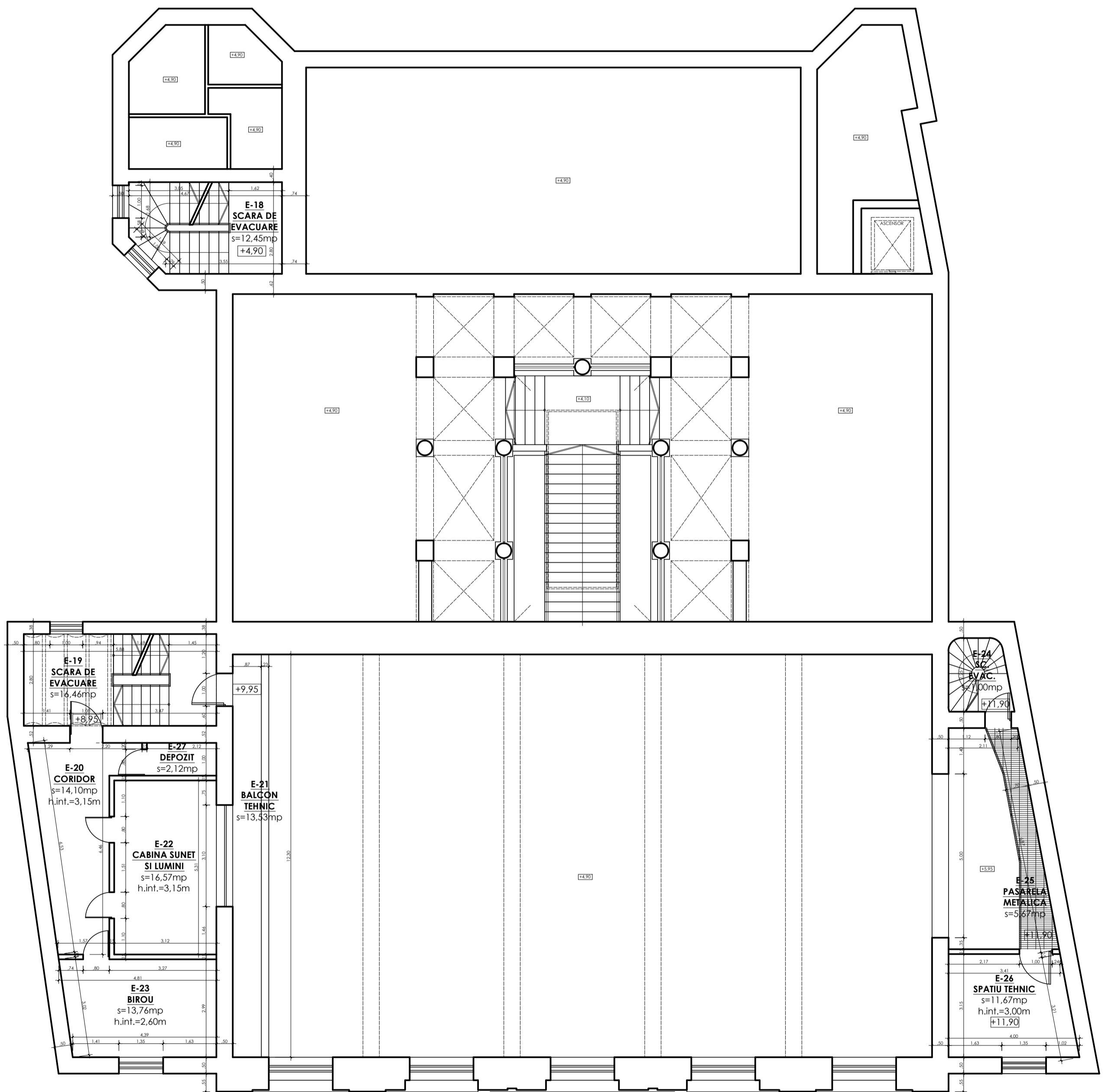
PLAN NIVEL INTERMEDIAR COTELE +8,95/+11,90 SITUATIA PROPUSA S.C.=194,23mp S.U. =107,33mp
